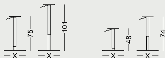
Con piastra 250x250 e blocchetto estetico With plate 250x250 and aesthetical join
